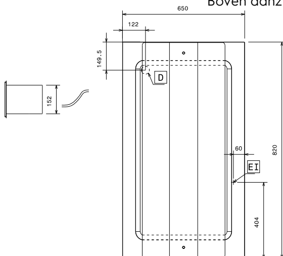
Boven aanzicht
