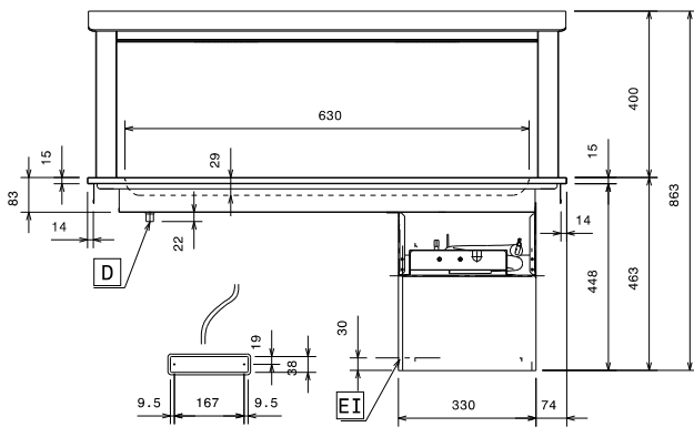
Zij aanzicht
